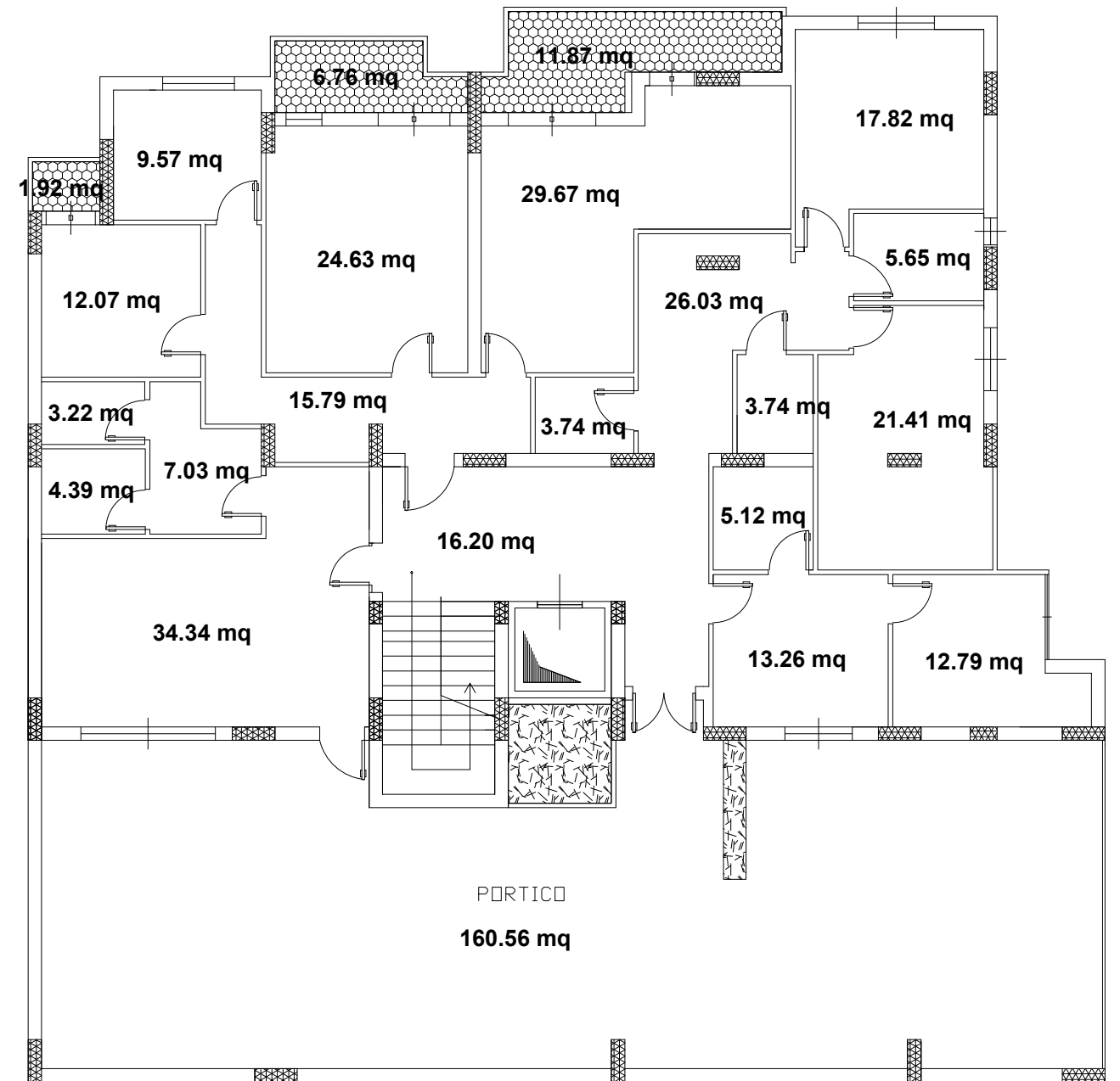
PIANO PRIMO
